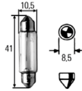
Festoon bulb 6 Volt, 5 Watt.
